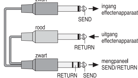
⑥ De aansluiting van de Y-kabel MCA-202 van MONACOR
