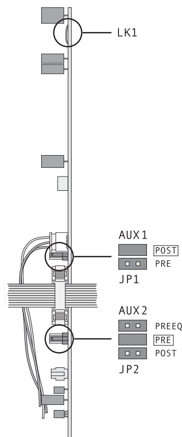
⑤ Circuito stampato di un canale d'ingresso
