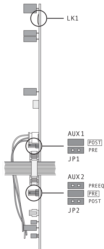
⑤ Circuit d'un canal d'entrée
